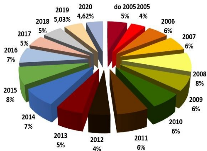
Dane w bazie AMRON (łącznie) w podziale na datę transakcji
