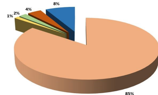
Dane pozabankowe w bazie AMRON w podziale na źródło informacji
