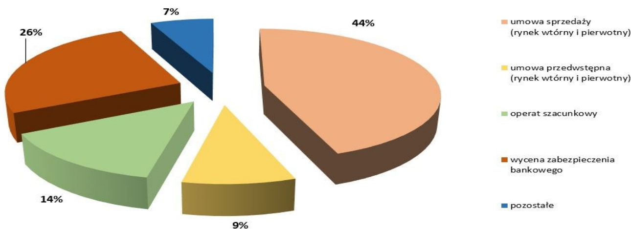
Dane bankowe w bazie AMRON w podziale na źródło informacji
